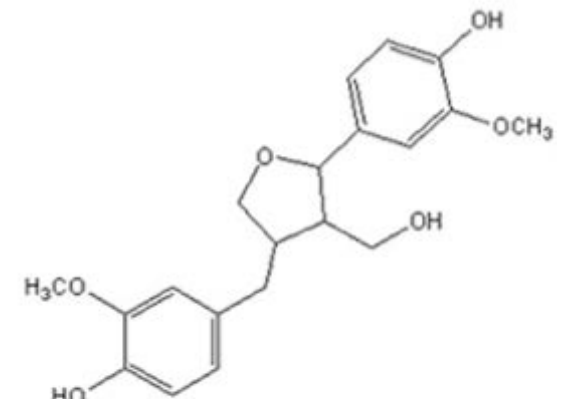
Lariciresinol
